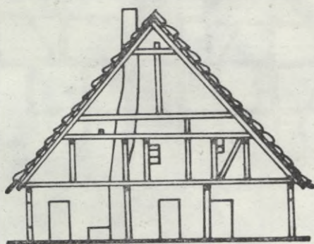
Ryc. 26. Dąbki, gm. Darłowo. Chatupa z zagrody nr 23. Wł. Edward Szymczyk. Rzut poddasza, przyziemia i przekrój poprzeczny
