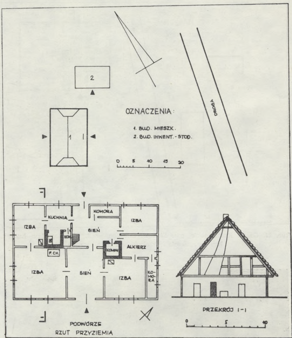
Ryc. 23. Bielkowo, gm. Sianów. Zagroda nr 33. Wł. Skarb Państwa. Plan zagrody, rzut przyziemia i przekrój chatupy
