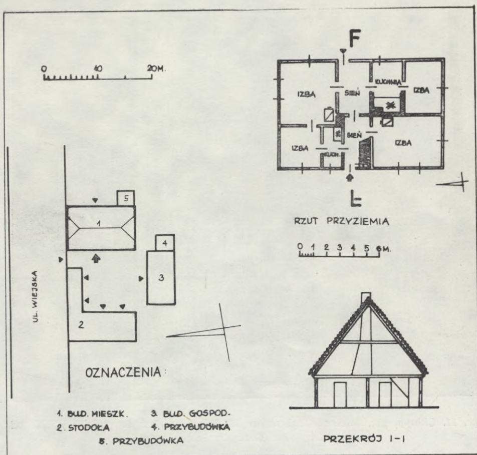
Ryc. 12. Chłopy, gm. Mielno. Chatupa nr 28. Wł. Stanisław Bargański. Rzut przyziemia, przekrój poprzeczny i plan zagrody
