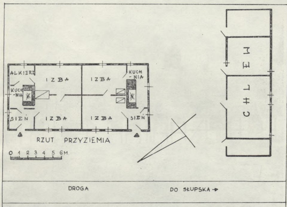
Ryc. 53. Kluki Smołdzińskie, gm. Smołdzino. Zagroda nr 2. Wł. Anna Kecz. Plan zagrody i rzut przyziemia chałupy
