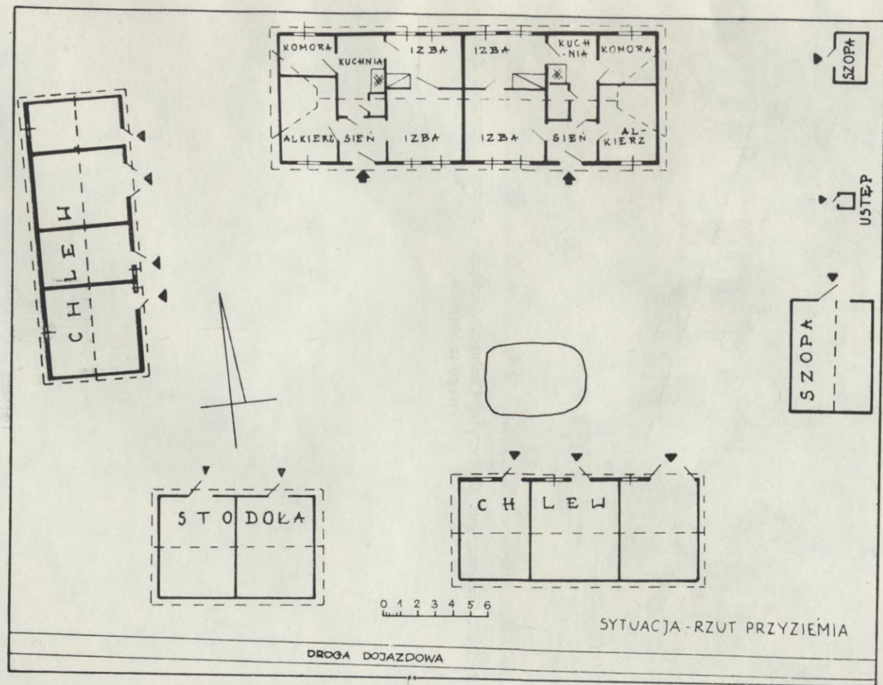
Ryc. 56. Kluki Zeleskie, gm. Smołdzino, Zagroda, nr 5. Wł. Skarb Państwa. Plan zagrody
