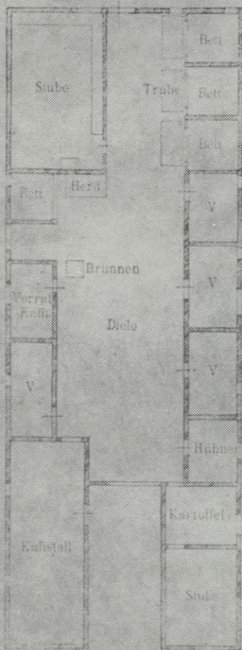
Abb. 2. Fischerhaus in Camp.
