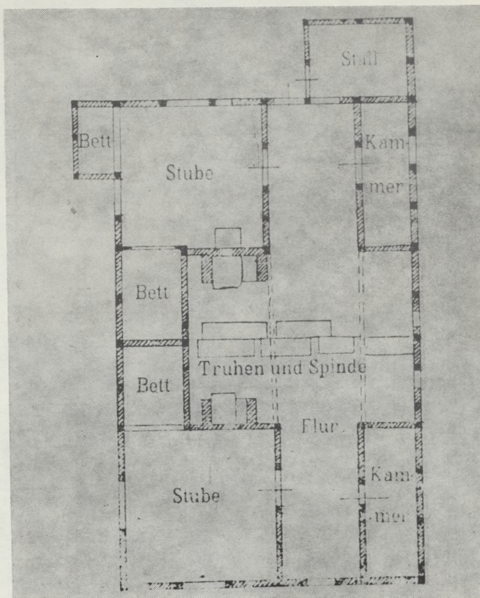
Ryc. 8. Ustronie Morskie, gm. Ustronie Morskie. Dwurodzinna chalupa Warnkego i Maassa. Wg B. Schmida
