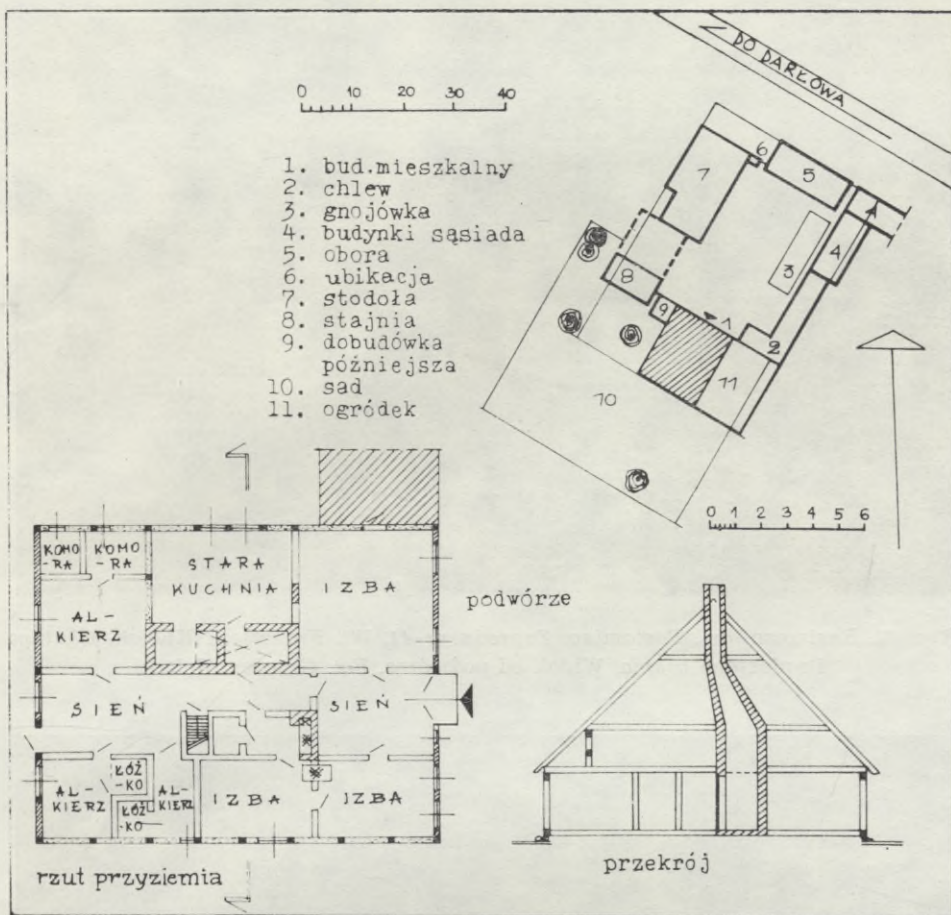
Ryc. 41. Krupy, gm. Dartowo. Zagroda nr 23. Wł. Henryk Kuś. Plan zagrody oraz rzut przyziemia i przekrój chatupy
