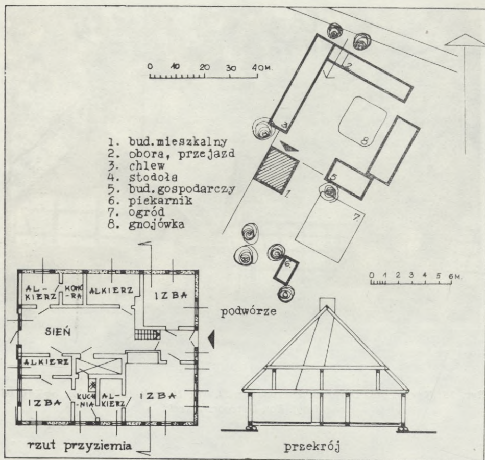
Ryc. 35. Krupy, gm. Darłowo. Zagroda nr 16. Wł. Antonina Szewczyk. Plan zagrody, rzut przyziemia i przekrój chałupy
