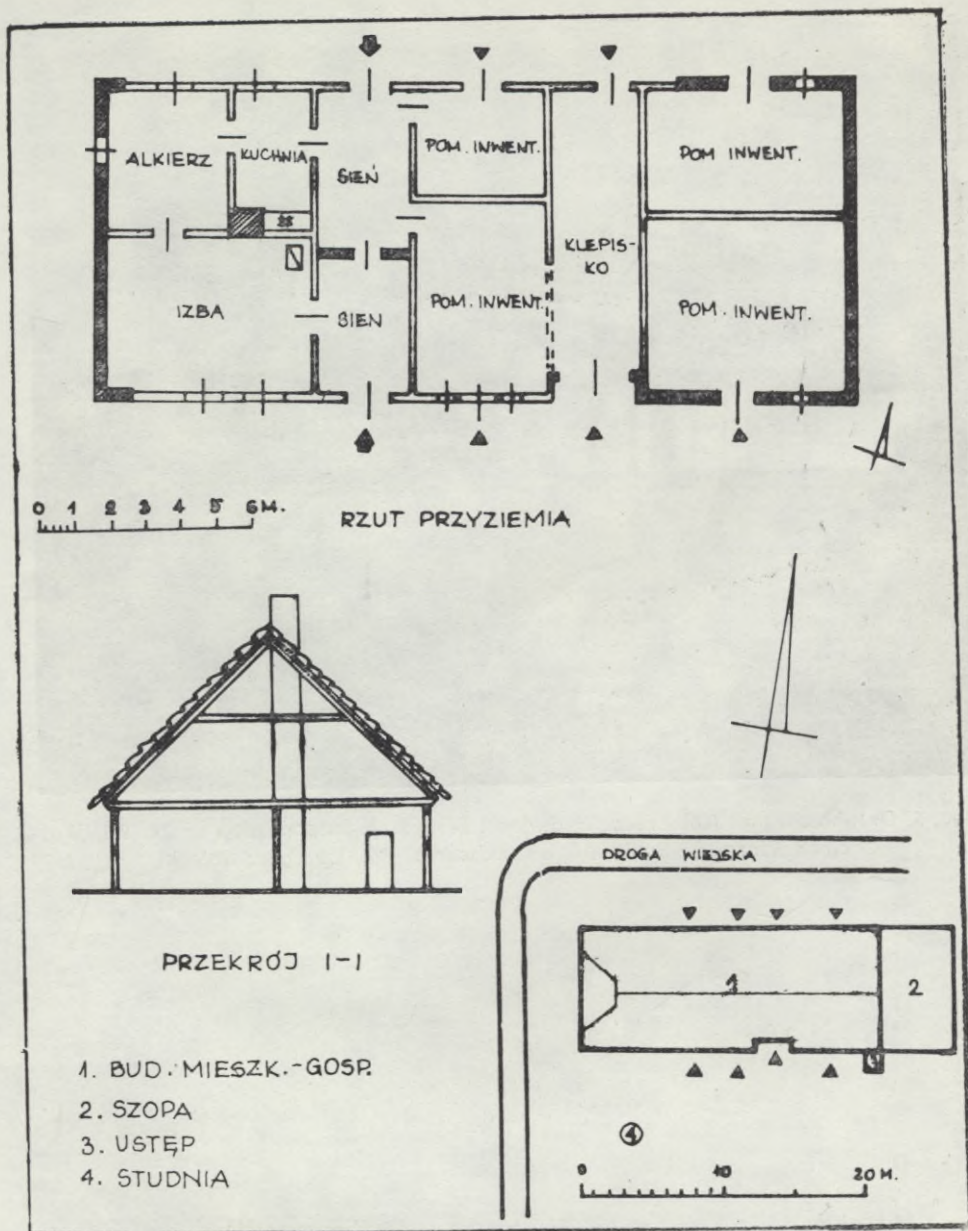
Ryc. 6. Grzybowo, gm. Kołobrzeg. Budynek mieszkalno-gospodarczy nr 28. Wł. Wojciech Szczęściwilk. Rzut przyziemia i przekrój oraz plan zagrody
