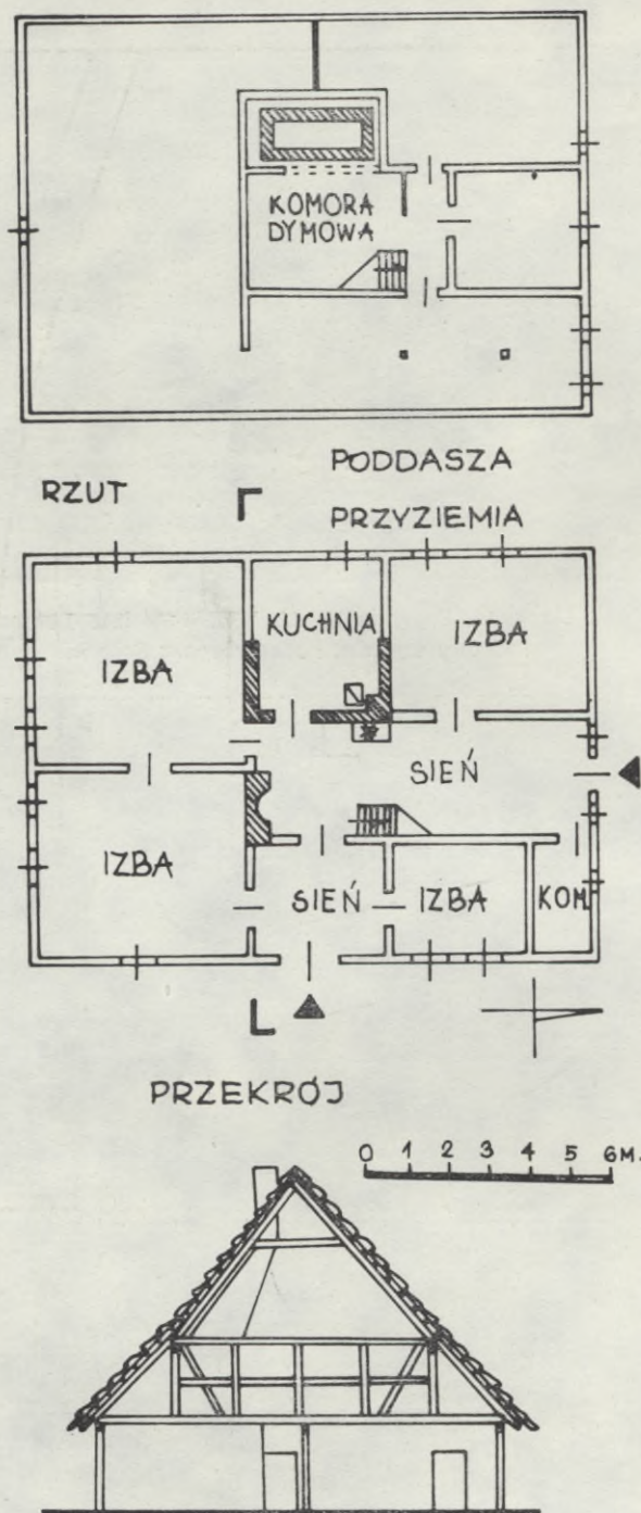
Ryc. 29. Dąbki, gm. Dariowo. Zagroda nr 18. Wł. Stanisław Lebioda. Rzut poddasza, przyziemia i przekrój poprzeczny
