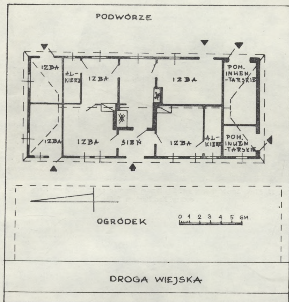
Ryc. 50. Rowy, gm. Objazda. Chałupa nr 17, słowińska. Wł. Kazimierz Piotrowski. Rzut przyziemia
