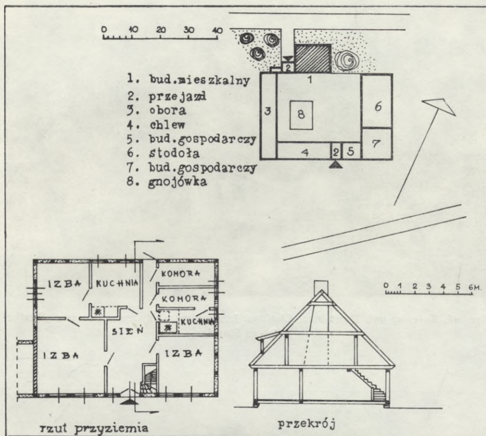
Ryc. 44. Rusinowo, gm. Postomino. Zagroda nr 41. Wł. Franciszek Kubiak. Plan zagrody oraz rzut przyziemia i przekrój poprzeczny chatupy
