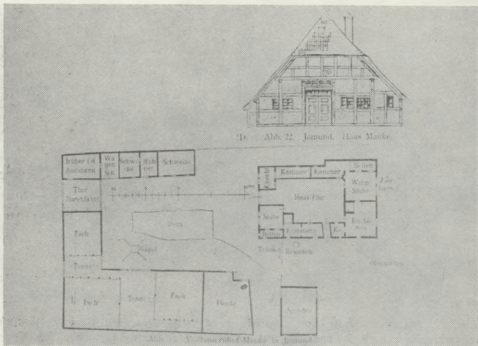
Ryc. 15. Jamno, gm. Będzino. Zagroda zamknięta Maukego. Wg B. Schmida
