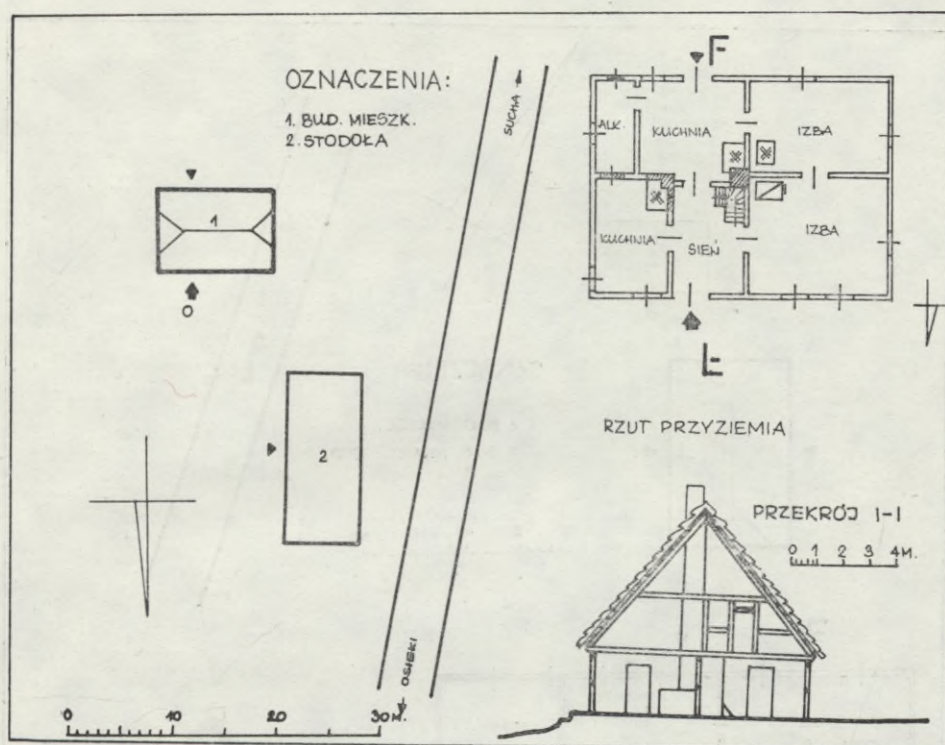
Ryc. 21. Osieki Koszalińskie, gm. Sianów. Chałupa nr 8. Wł. Bogusław Łuczak. Rzut przyziemia i przekrój oraz plan zagrody
