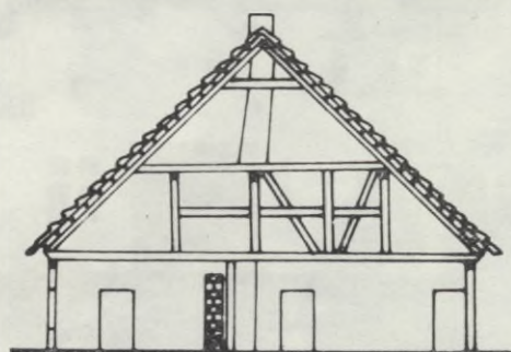
Ryc. 32. Dąbki, gm. Darłowo. Chałupa z zagrody nr 21. Wł. Anna Mielniczek. Rzut poddasza, przyziemia i przekrój poprzeczny
