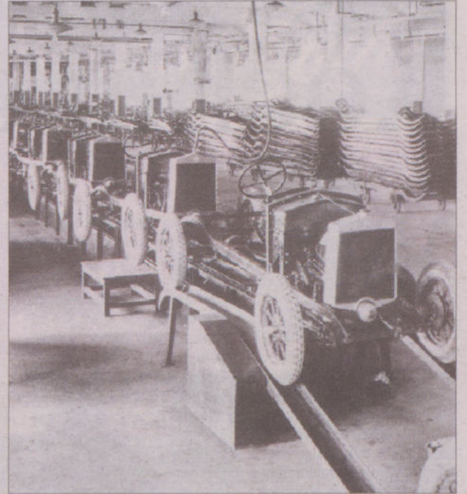
Taśma produkcyjna w Lingotto. Podwozia modelu 509 wyposażano w zabudowy bądź w macierzystej fabryce, bądź w specjalistycznych firmach karoseryjnych.
