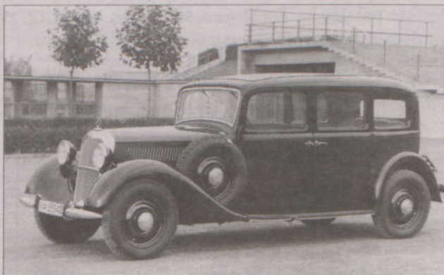
Pierwszy samochód osobowy z silnikiem wysokoprężnym Mercedes-Benz 260D wyprodukowano w 1936 r. Napędzany był 4-cylindrowym silnikiem 2.6 l o mocy 45 KM.
