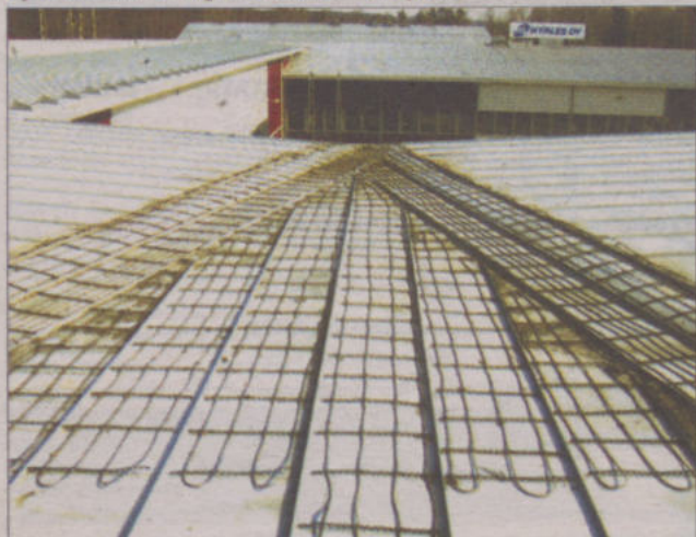
System podgrzewania dachów płaskich.
