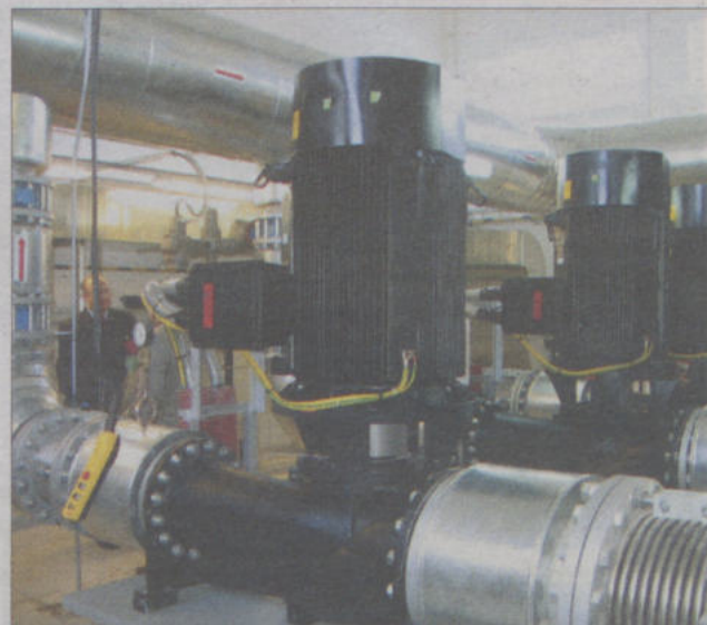
Nowe pompy do podnoszenia ciśnienia w sieci dostarczającej ciepło do południowych dzielnic Gdańska. Zbudowało je GPEC, przy ul. Grota Roweckiego i Ciasnej w Gdańsku.
