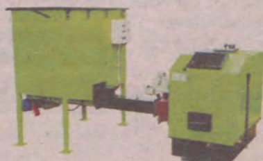
zestaw: SMOK II i kocioł 50 kW
