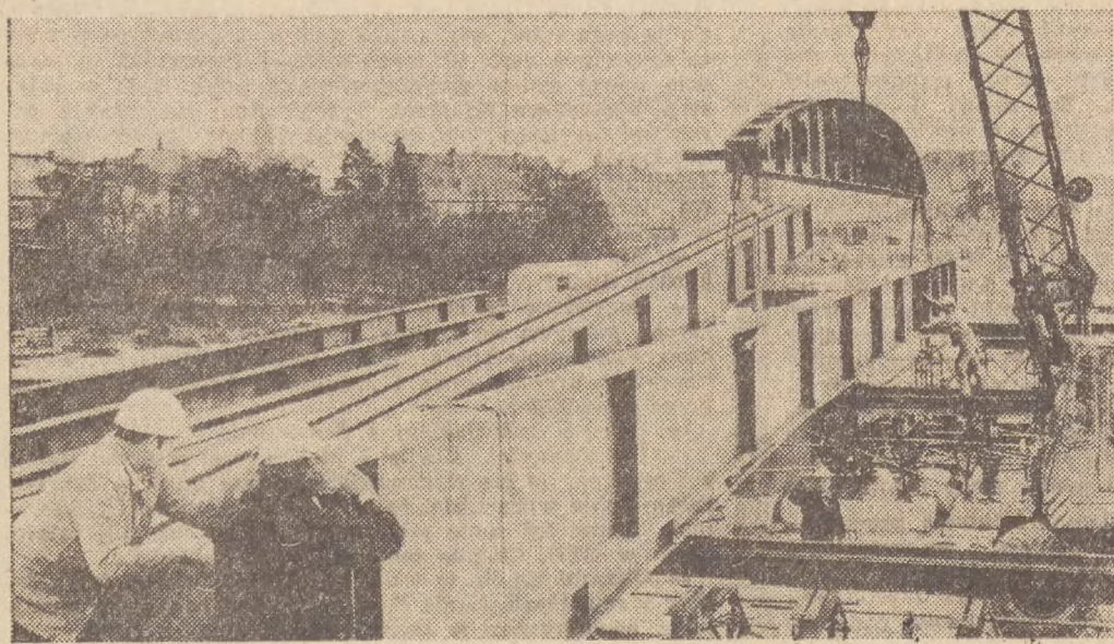
Waren, nad zsiorem Müritz, to znana i licznie odwiedzana miejscowość wypoczynkowa. Obecnie buduje się tu nowoczesny węzeł komunikacyjny, w tym (na zdjęciu) kilka mostów. Ważna to budowa, zważywszy że aktualnie do 12 godzin na dobę opuszczane tu bywają szlabany kolejowe.
