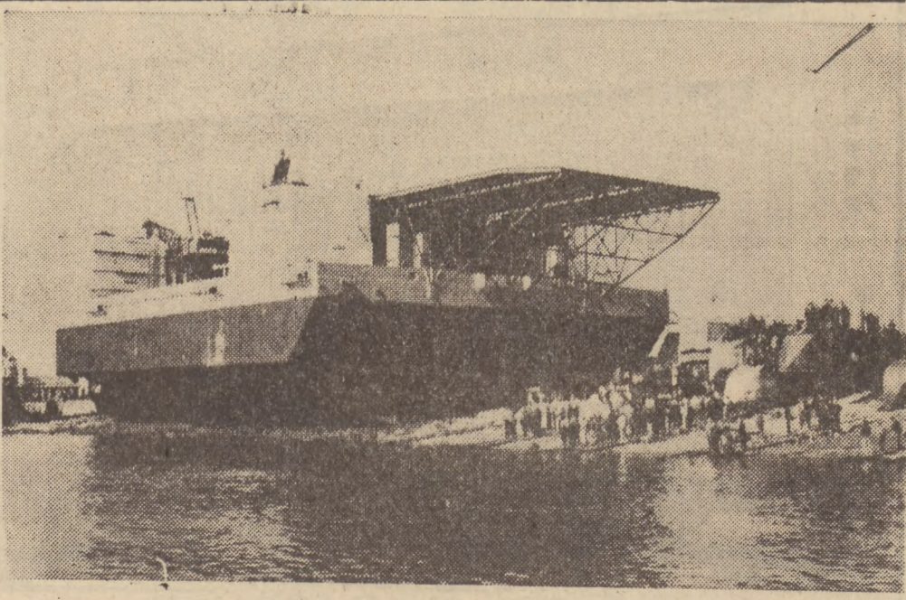
W stoczni w Galaży zbudowano pierwszą zbudowaną w Rumunii pływającą platformę wiertniczą „Gloria”. Wysokość urządzenia łącznie z wieżą wiertniczą wynosi 70 m nad poziomem morza, szerokość 41 m, długość 52 m. Platforma o łącznej wadze wraz z urządzeniami 6800 ton spoczywać będzie na 122-metrowych czterech betonowych słupach. Jest ona przeznaczona do podwodnych wierceń u wybrzeży Morza Czarnego. Na zdjęciu: pierwsza rumuńska platforma pływająca przed wodowaniem.
