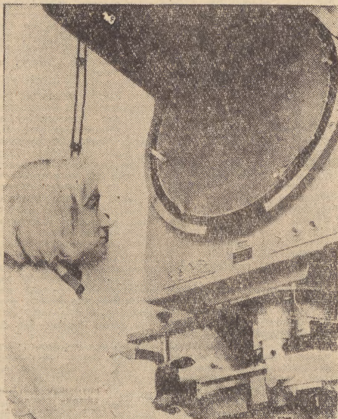
Wydział P-6 koszalińskiego Ośrodka Naukowo-Produkcyjnego Materiałów Półprzewodnikowych. Przy projektorze kontrolnym Wanda Kurylowicz, wyróżniona ostatnio w wojewódzkim współzawodnictwie odznaką Przewodnika Czynu Zjazdowego, dokonuje pomiaru sitek do sokowirówek, przeznaczonych dla zakładów „Predom” w Skarżysku-Kamiennym.
