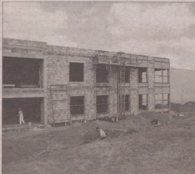
Trwają ostatnie prace przy budowie hali.
