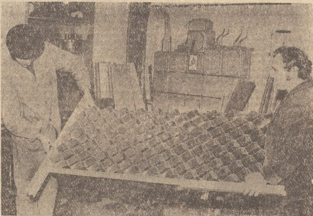
W oprzyrządowaniu zakładowej wykonuje się także prototypy nowo wprowadzanych do produkcji elementów konstrukcyjnych, urządzeń i mebli. Przy nowo zaprojektowanych elementach lekkiego podwieszanego stropu do pawilonów S-400 pracownicy ZPIUT, Tadeusz Sagan i Roman Czulewicz.
