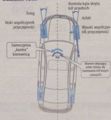
Tak działa VDIM w nowym Lexusie GS 430. Zależnie od przyczepności poszczególnych kół podczas hamowania oraz ich ustawienia, system koryguje siłę hamowania każdego z kół oraz wykonuje „kontry” kierownicę.
