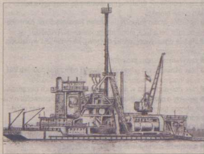
Asfalcjarka, statek do układania asfaltu na dnie różnych budowli wodnych.
