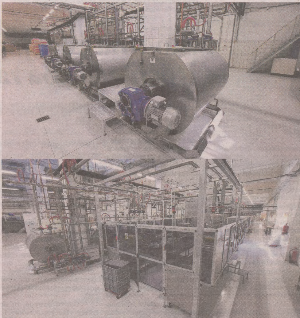
Linia formowania wyrobów czekoladowych
