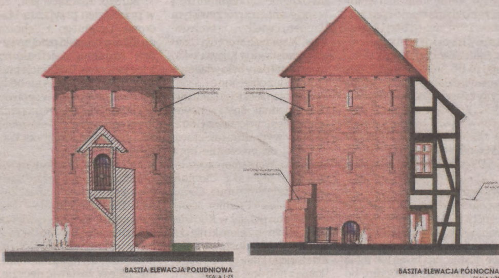
BASZTA ELEWACJA POŁUDNIOWA SKALA 1:75
