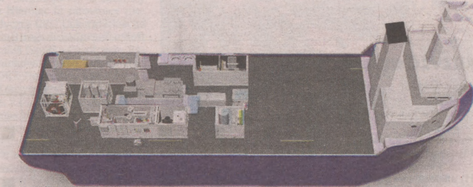
System do utylizacji broni chemicznej ma być posadowiony w kontenerach na statku
