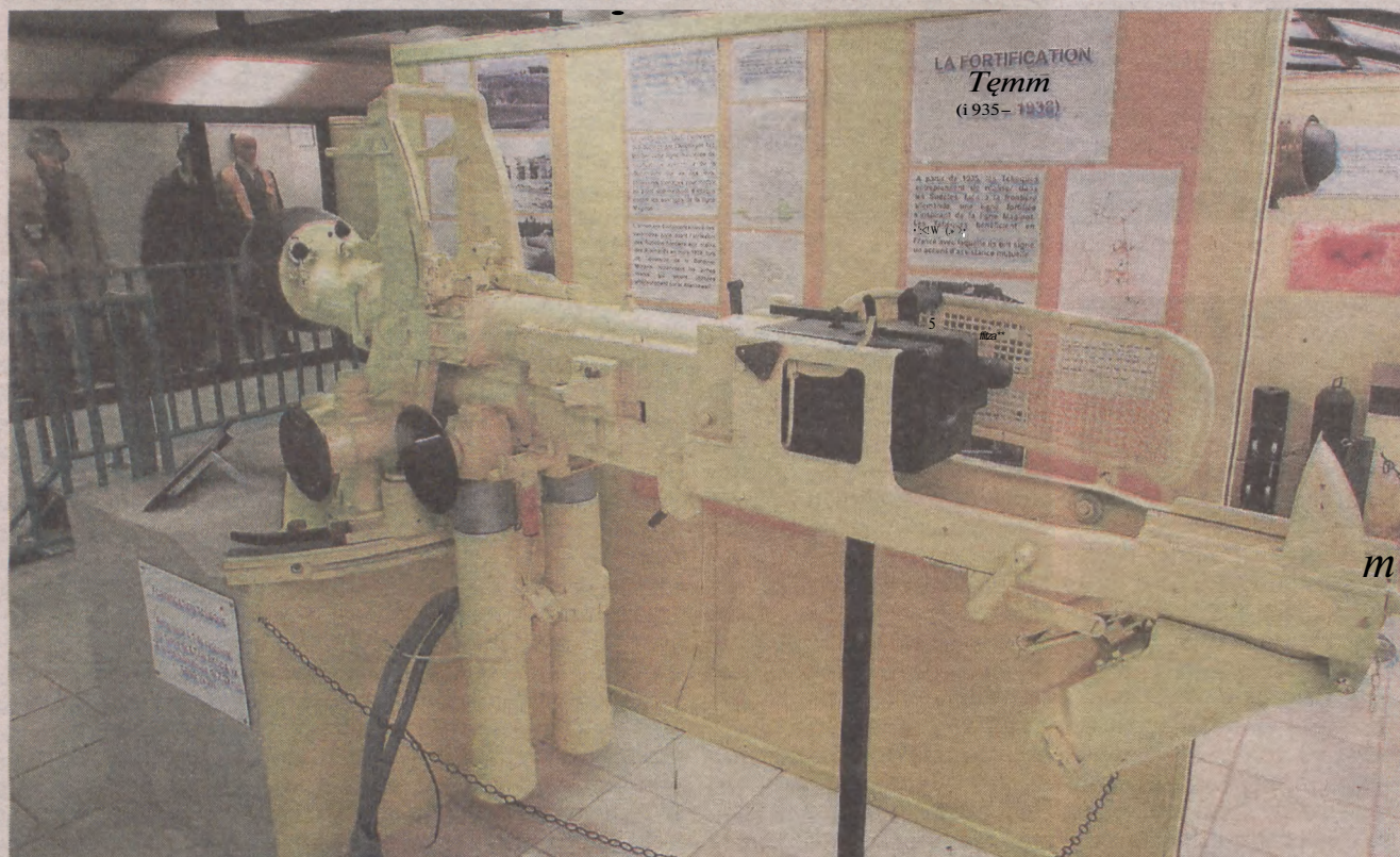
Ekspozycja w fort de Fermont. Czeska armata Skoda Vz 36 4,7cm (podobna była w szczecińskiej ścianie) sprzężona z karabinem 7,92mm Brno Vz 37
