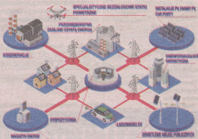
Rys. Przykładowy schemat mikrosieci w samorządzie
