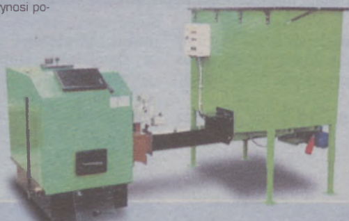
W skład systemowego rozwiązania przeznaczanego do spalania odpadów drzewnych wchodzi: urządzenie o nazwie „Smok” i kocioł Moderator.
