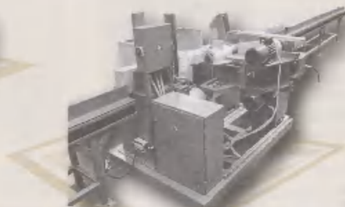
Фрейзерный четырехсторонний станок с функцией сверления тип DFPR-250.
