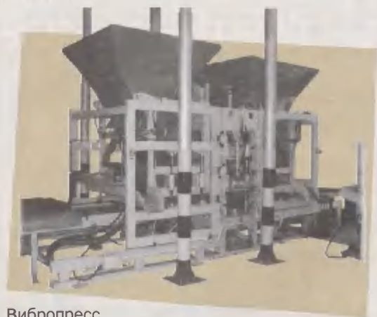
Вибропресс
