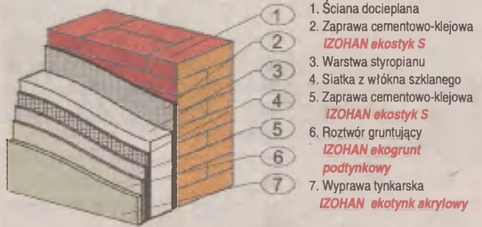
Elewacja SP we Wrześni k. Słupska w systemie IZOHAN
