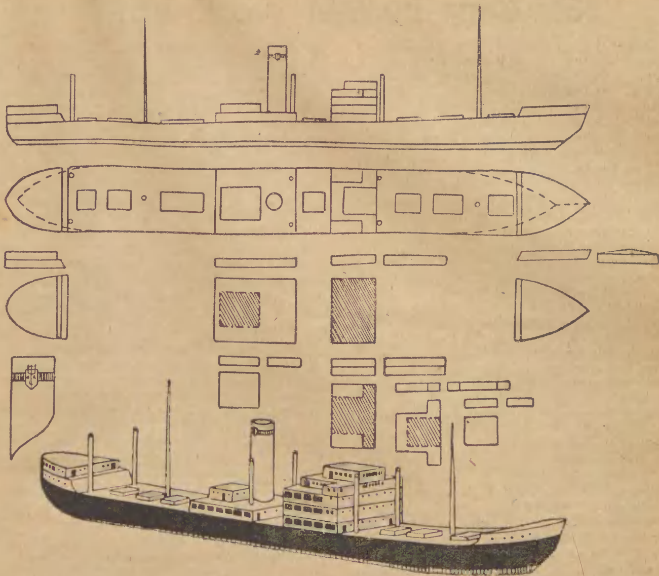
Rysunki modelu parowca drobniczego
