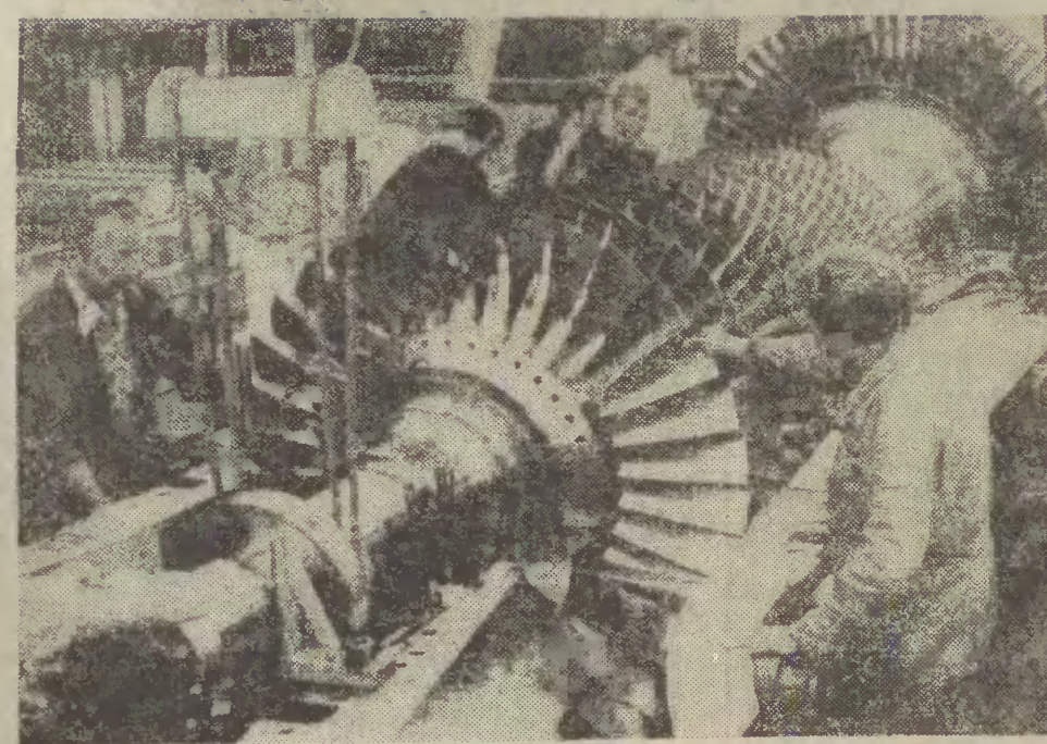
Turbina gazowa w końcowej fazie montażu.
