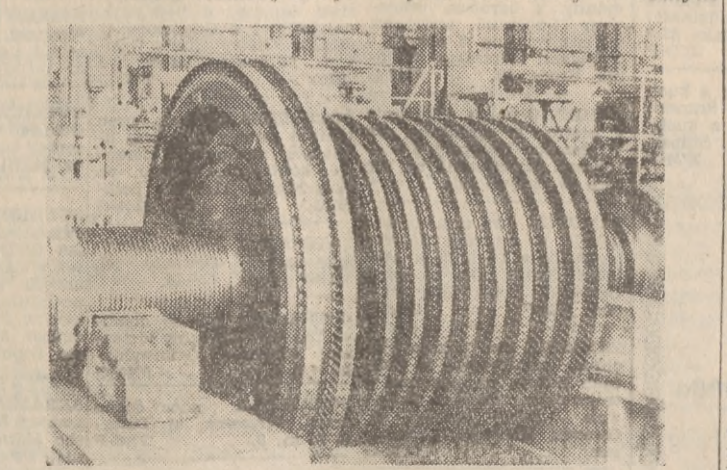
Na zdjęciu: wirnik turbiny TP-2. Produkcja tych turbin, po przeprowadzeniu pierwszych prób, ma już dziś charakter seryjny.
